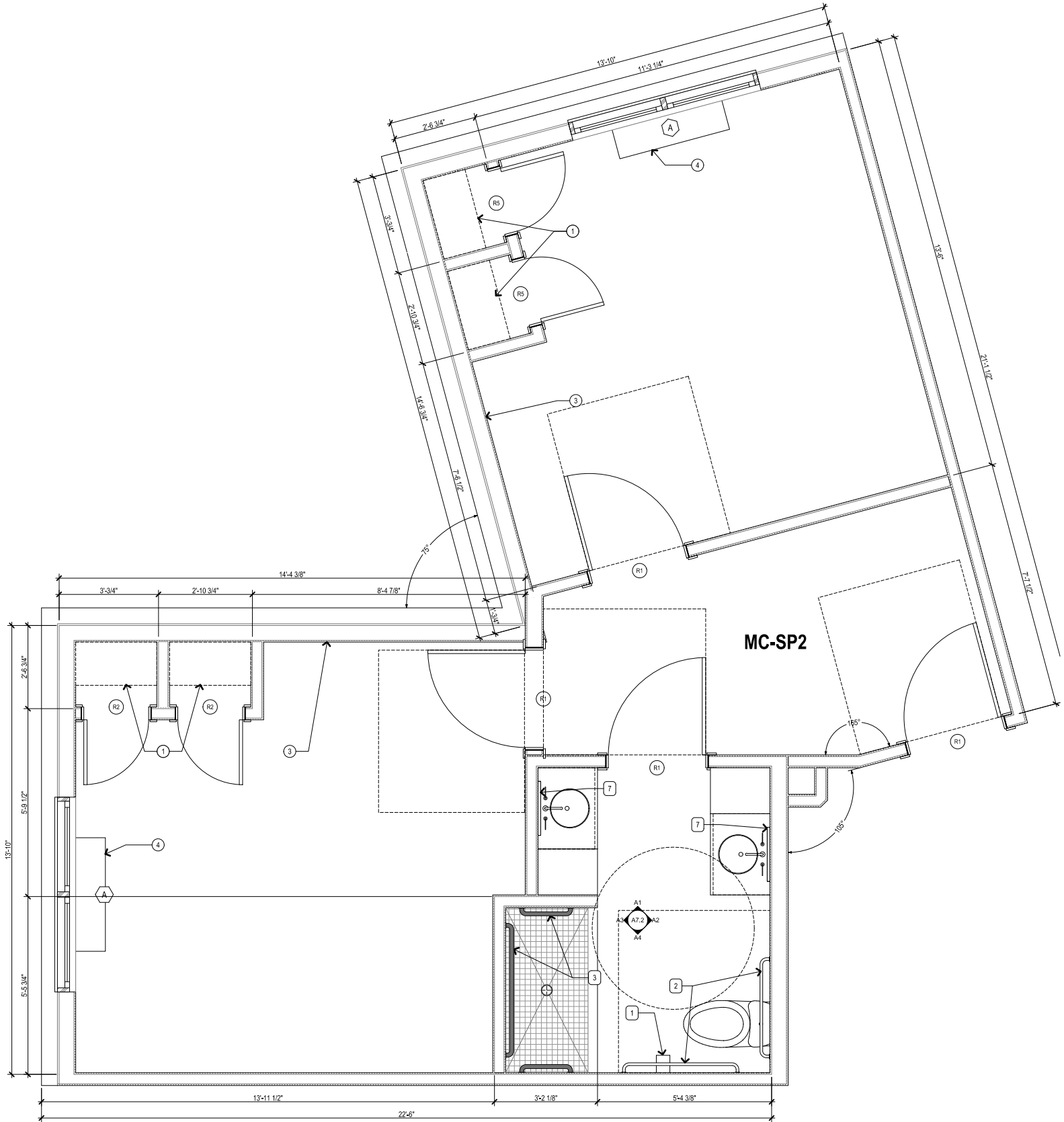
A3 TYP. MC-SP2 SCALE: 1/2" = 1'-0"
